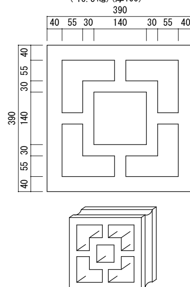
二重角型 開口率 40.0% Y. D-4-1 (16.5 kg) (厚100)
