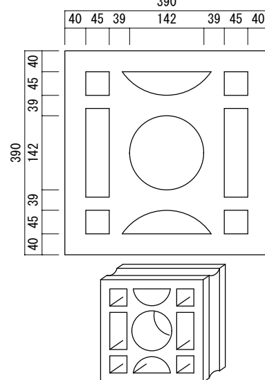
角丸型 Y. D-2-1 (17.0 kg) (厚100)
