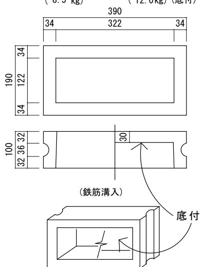
角型(Aフラット) Y. C-4-3 (8.5 kg) Y. C-4-4 (12.0 kg) (底付)
