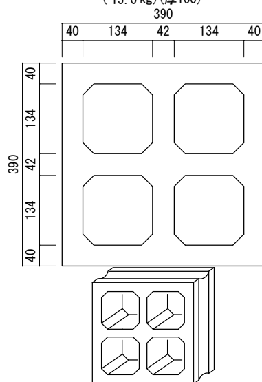
十字型 開口率 44.6% Y. D-3-1 (15.0 kg) (厚100)
