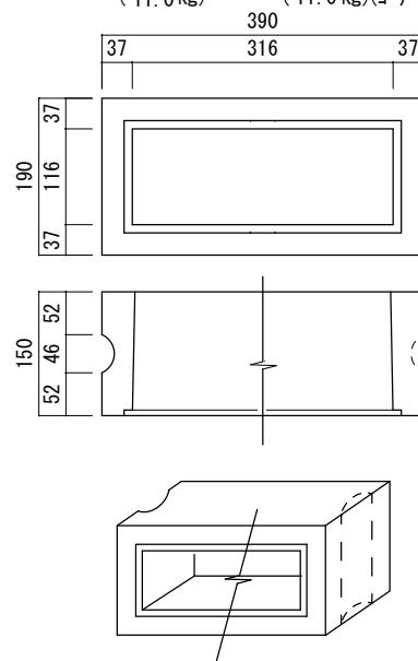
角型(大) Y. C-6-1 (11.0 kg) Y. C-6-2 (11.0 kg) (コナ-)
