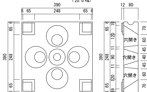
M-4 内井昭蔵建築設計事務所 ( 20.0 kg) 内井昭蔵氏 作品
