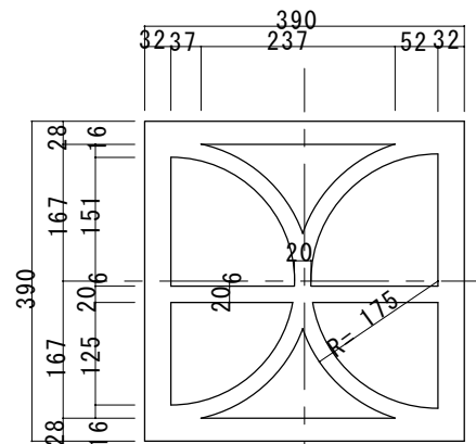
三方鉄筋ミゾ有り
