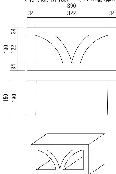
角型(Cタイプ) 角型(Dタイプ) Y. C-7-1 (13.2 kg) (厚150) Y. C-7-2 (15.5 kg) (厚190)
