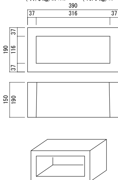
角型(Bタイプ) Y. C-5-1 (11.0 kg) (厚150) Y. C-5-2 (16.0 kg) (厚190)
