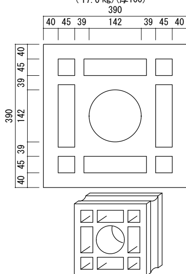
角丸型 Y. D-2-2 (17.0 kg) (厚100)
