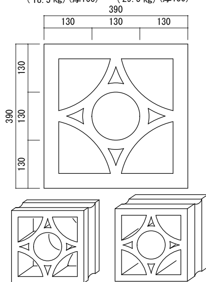
角丸三日月型 (大) 開口率 Y. D-1-1 (18.5 kg) (厚100) Y. D-1-2 (29.5 kg) (厚150) 32.8%
