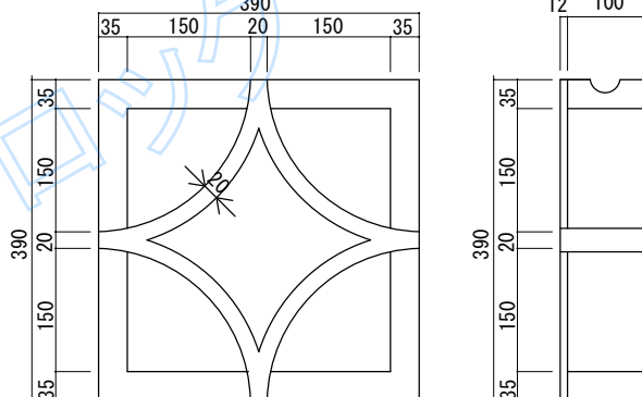
星 H-2 参考重量 15 kg 厚100 x 390 x 390 開口率 55.44%
