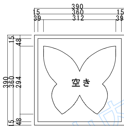
蝶 重量 = 15kg 厚100 x 390 x 390 B-1
