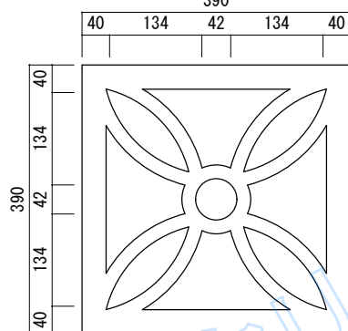
花 H-1 参考重量 16.5kg 厚100 x 390 x 390 開口率 40.48%
