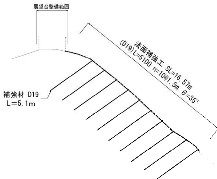
法面整形
