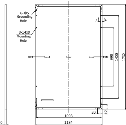
背面図 (mm)
