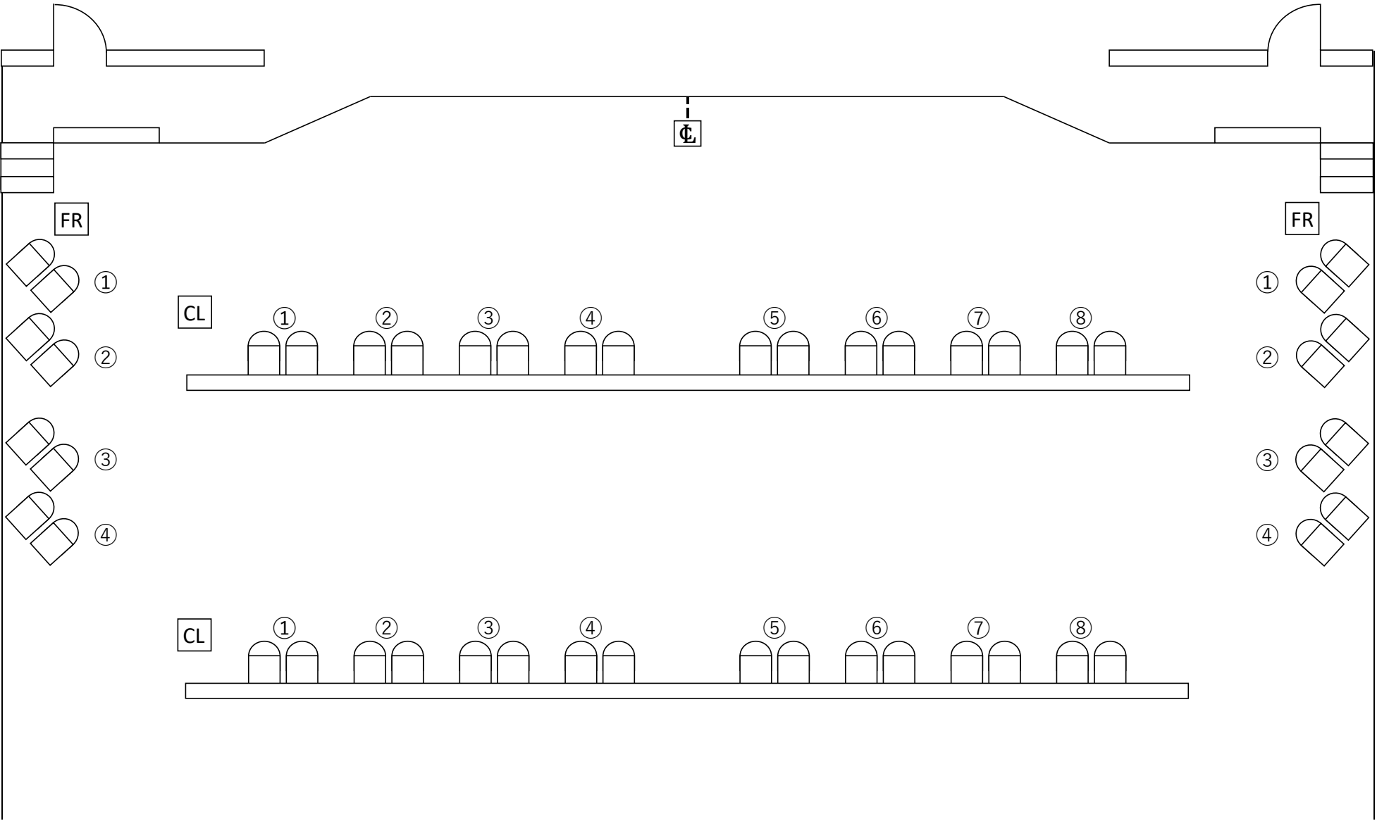
さわふじ未来ホール（客席照明仕込み図）
