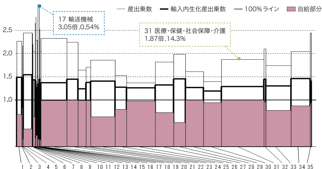
図 沖縄県産業連関表(令和2年)のスカイラインチャート(縦軸：倍率、横軸%)
