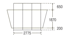
天幕(平面図)
