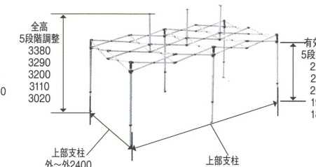
フレーム
