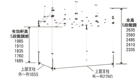
フレーム
