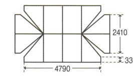
天幕(平面図)
