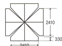
天幕(平面図)
