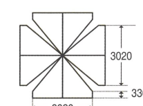
天幕(平面図)
