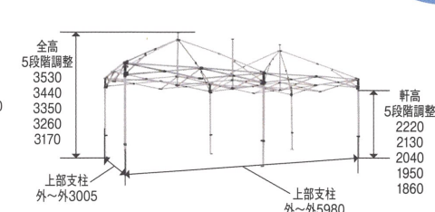
フレーム
