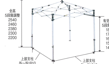
フレーム
