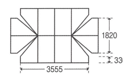
天幕(平面図)
