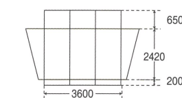
天幕(平面図)
