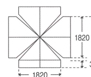
天幕(平面図)
