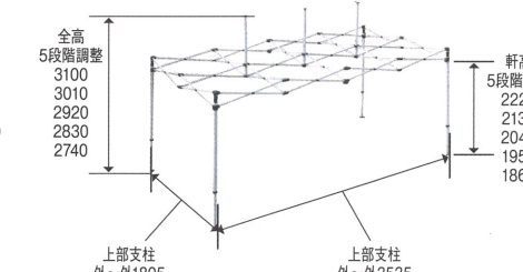
フレーム
