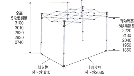
フレーム
