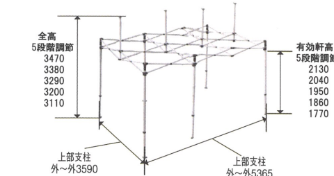
フレーム
