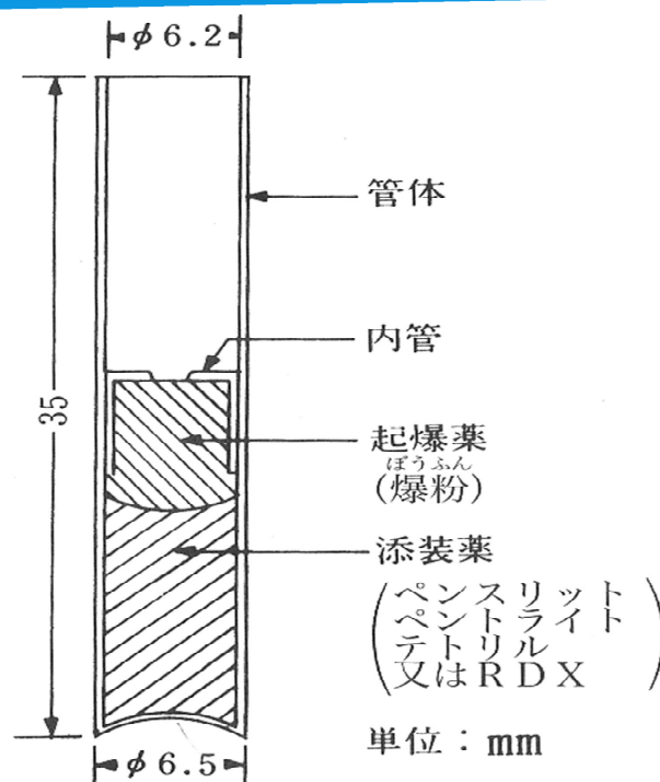
第 4.2 図 工業雷管断面図
