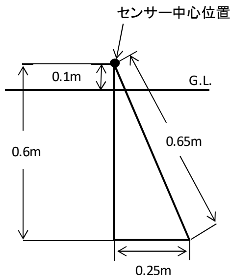
センサーからの位置関係 (5 インチ砲弾仕様の場合)
